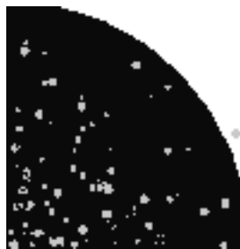
mapalgebra intersektion
