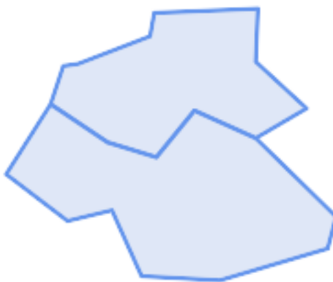
Originalgeometrier
