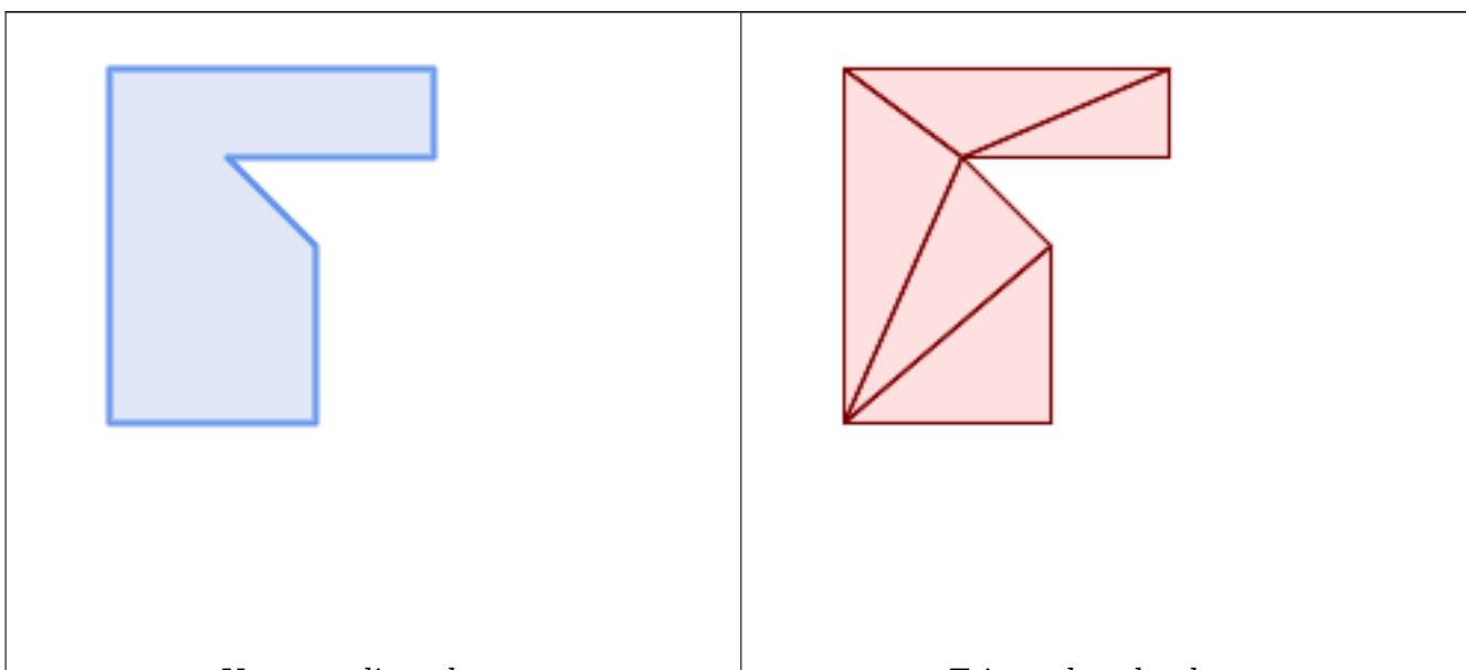
Ursprunglig polygon
