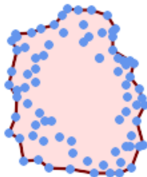
Forme alpha d'un multipoint (même exemple que ST_OptimalAlphaShape )
