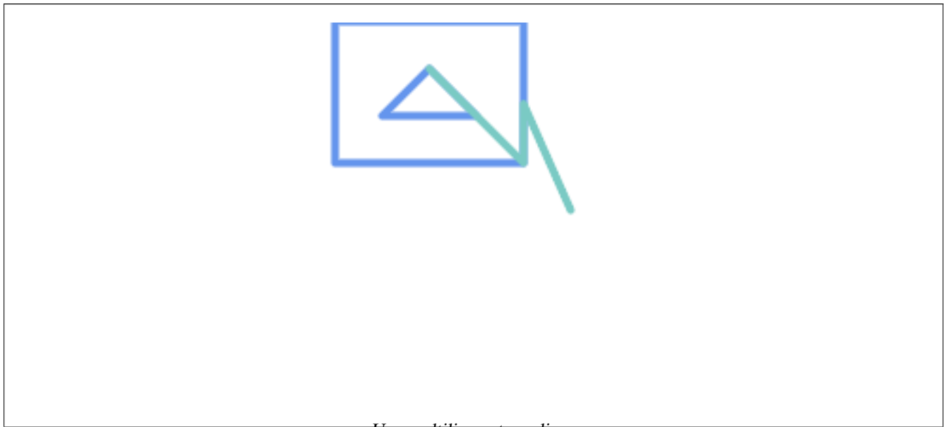
Une multiligne et une ligne
