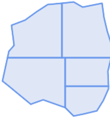
Subdivisé en un maximum de 10 sommets
