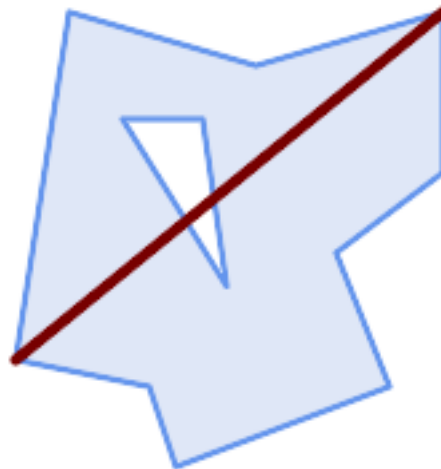
Ligne la plus longue traversant une seule géométrie. La longueur de la ligne est égale à la distance maximale. Les extrémités de la ligne sont situées sur le cercle de délimitation minimal.
