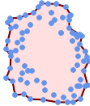
Forme alpha optimale d'un MultiPoint (même exemple que ST_AlphaShape )
