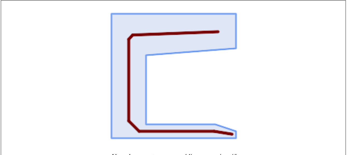
Un polygone et son axe médian approximatif
