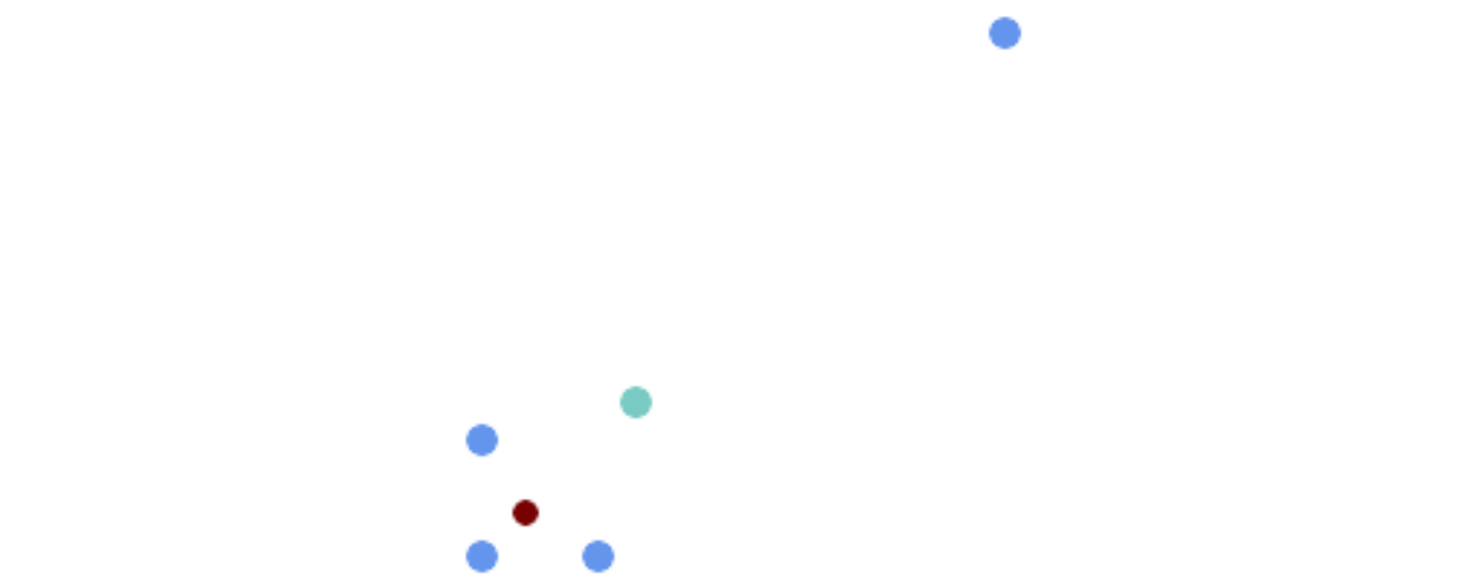
Comparaison de la médiane géométrique (rouge) et du centroïde (turquoise) d'un MultiPoint.
