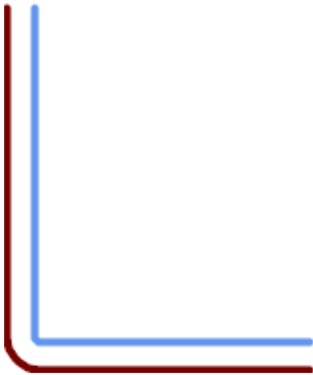
15, 'quad_segs=4 join=round' ligne originale et son décalage de 15 unités.
