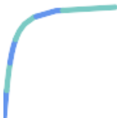
Les lignes densifiées et divisées.
