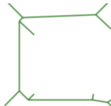
Squelette d'un polygone
