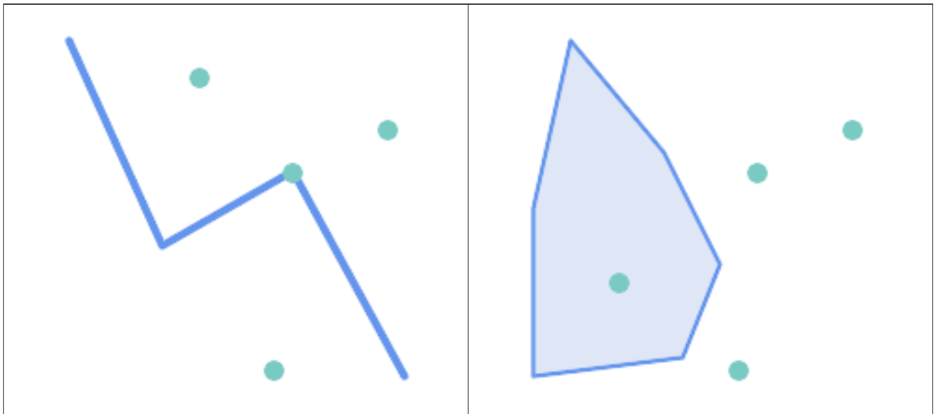
MEHRPUNKT / LINESTRING
