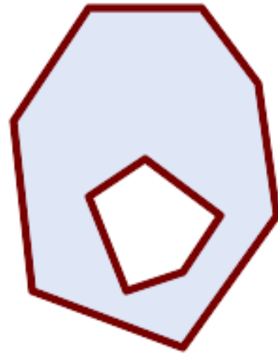
Polygon mit Lücke und der Abgrenzung/Boundary als Multilinestring
