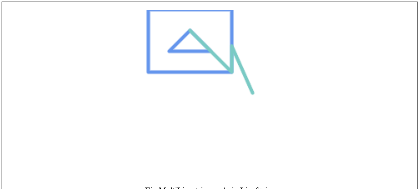
Ein MultiLineString und ein LineString
