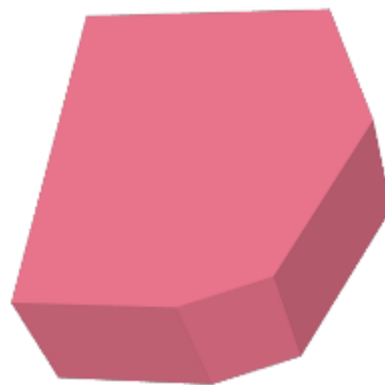
geom1 和 geom2 的交集
