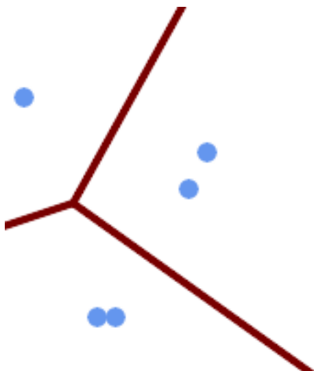
Voronoi 图，容差 30 个单位
