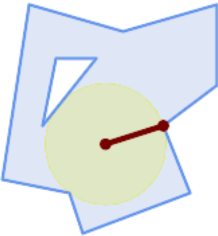
多边形形的最大内切圆。返回中心、最近点和半径。
