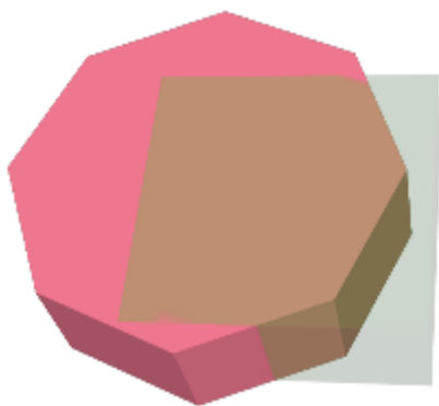
原始 3D 几何体相加。geom2 显示半透明
