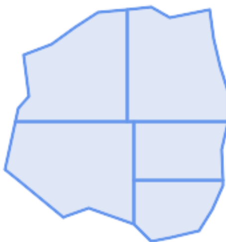
分至最多 10 个点
