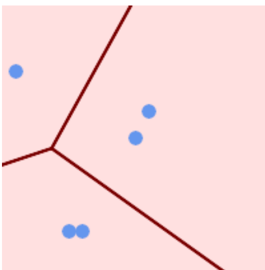
Voronoi 图，容差 30 个单位
