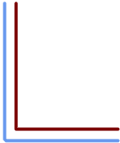
-15、'quad_segs=4 join=round' 原始图及其偏移量-15 个单位
