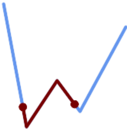
在 1/3 中范围上添加的 LineString (0.333, 0.666)
