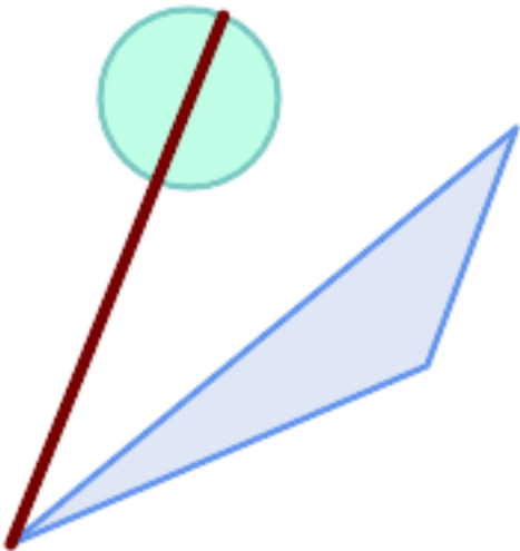
一个多边形之间最长的线
