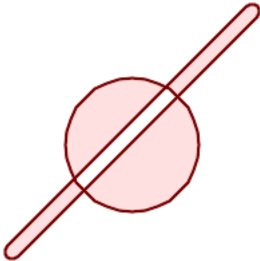
after_geom : 具有四个非重叠多边形的多多边形
