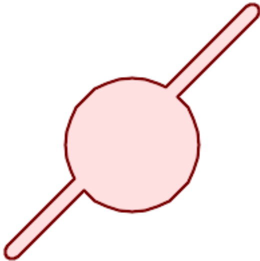
after_geom_structure : 由四个非重叠多边形形成的多多边形
