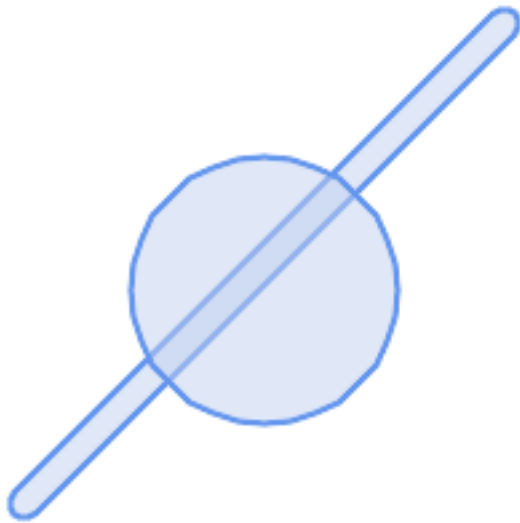
before_geom : 由一个重叠多边形形成的多多边形
