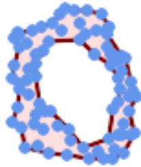
Forme alpha d'un MultiPoint, autorisant les trous (même exemple que ST_OptimalAlphaShape )
