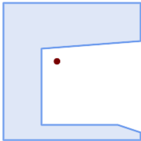
Geometrischer Schwerpunkt eines POLYGON
