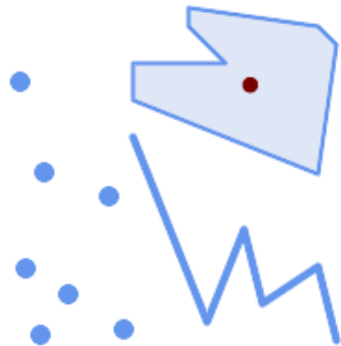
Der geometrische Schwerpunkt einer GEOMETRYCOLLECTION
