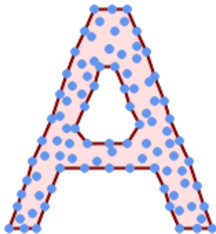
Konvexe Hülle eines MultiLineString und eines MultiPoint
