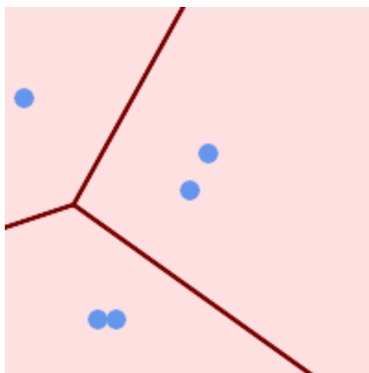
許容距離 30 単位のボロノイ図
