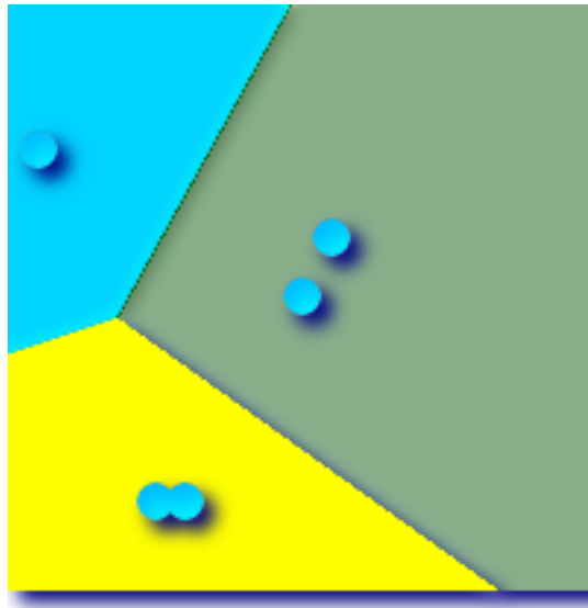
Voronoi mit einer Toleranz von 30 Einheiten
