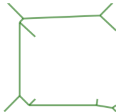
Das "Gerippe" des Polygons
