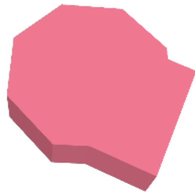
Vereinigung von geom1 und geom2
